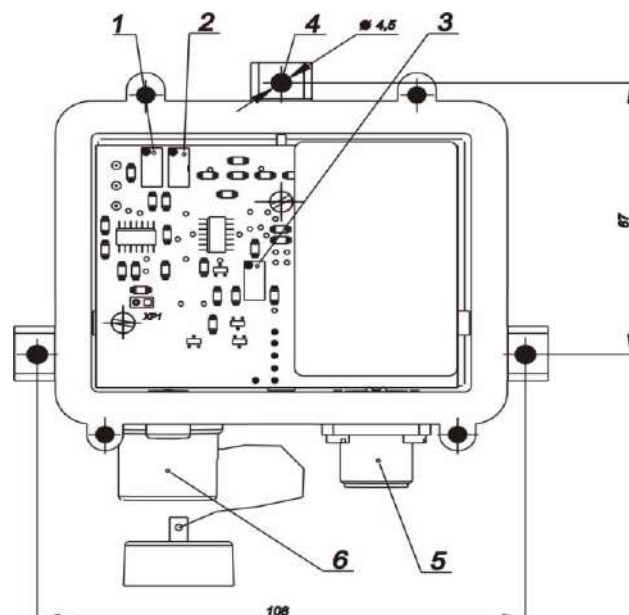
Рис.3.Датчик СИГМА-03.ДВ со снятой крышкой, присоединительные размеры. 1-потенциометр балансировки моста, 2-потенциометр регулировки начального тока, 3- потенциометр регулировки усиления, 4 – ,установочные отверстия диаметром 4.5 мм, 5 –розетка питания 6 – сенсор.
